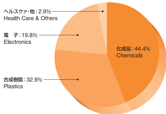
化学品 Chemicals
