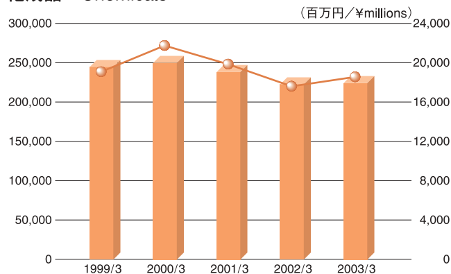
化学品 Chemicals
