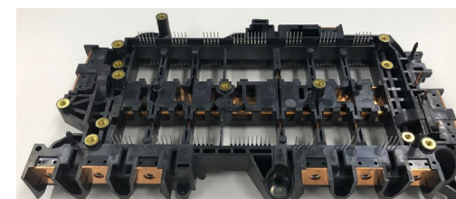
車載インバーター用金属インサート成型部品
